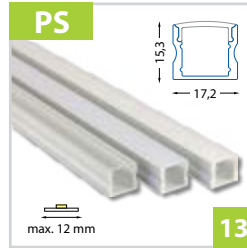
Přisazený hliníkový profil 17x15 mm - pro pásy do šíře 12 mm
